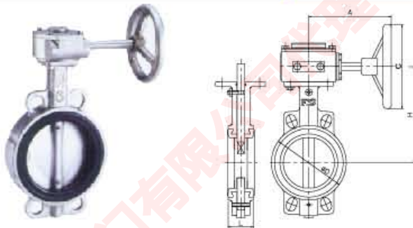
單位/mm
