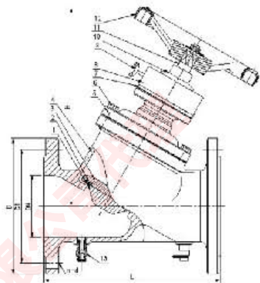
结构图
