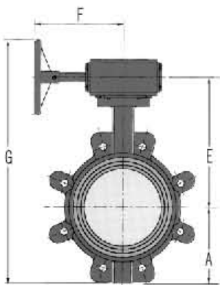
FIG: FS046 齒輪式
