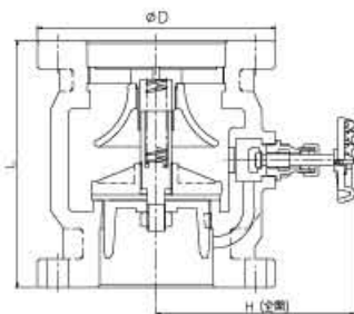
單位/mm
