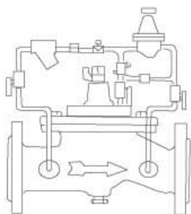
FIG: FS200X 減壓閥
