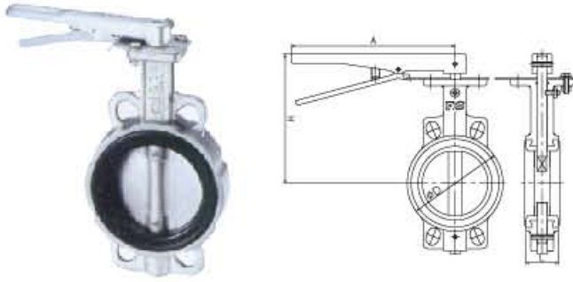
單位/mm
