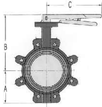
FIG: FS045 把手式
